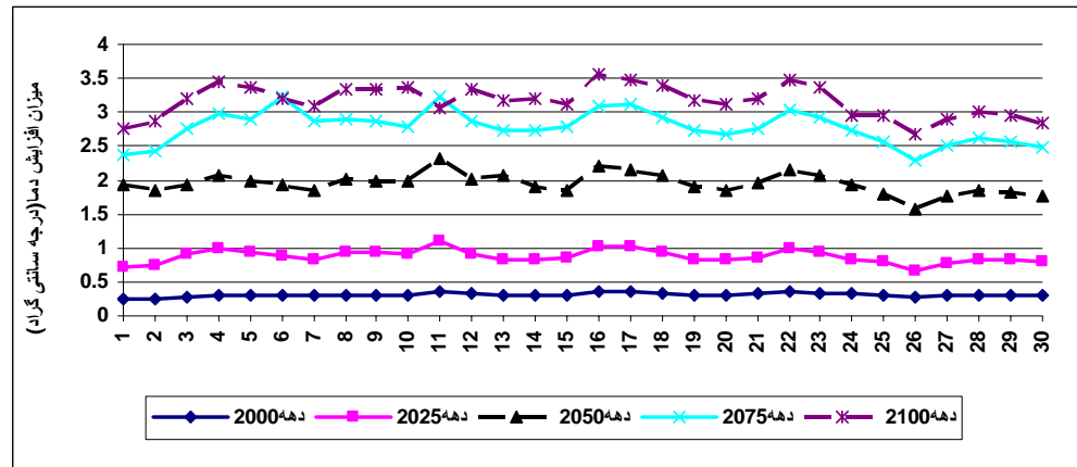
شکل ۳: میزان افزایش دما در مناطق ۳۰ گانه ایران طبق سناریوی WRE450
