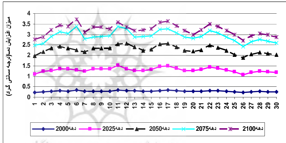
شکل ۴: میزان افزایش دما در مناطق ۳۰ گانه ایران طبق سناریوی B1MES
