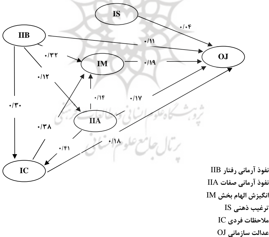
شکل ۱. شکل مسیر پیش بینی عدالت سازمانی از روی مؤلفه های رهبری تحول آفرین
