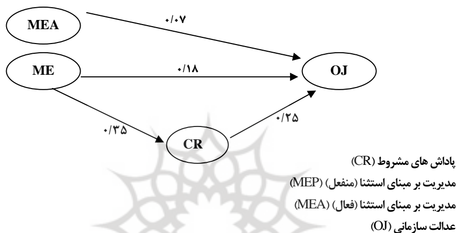
شکل ۲. نمودار مسیر پیش بینی عدالت سازمانی از روی مؤلفه های رهبری تبادلی
