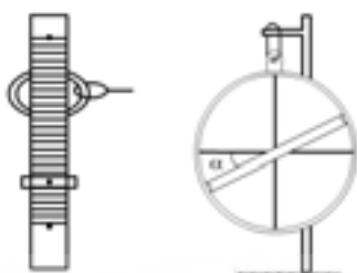
شکل ۸- تراز دوربینی کرجی (کرجی، ص ۱۲۳)
