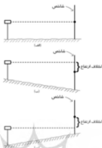
شکل ۱۳- سه حالت تراز و شاخص نسبت به یکدیگر
