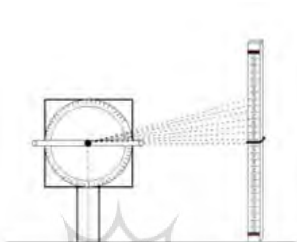
شکل ۱۵- مدرج کردن تراز دوربینی
