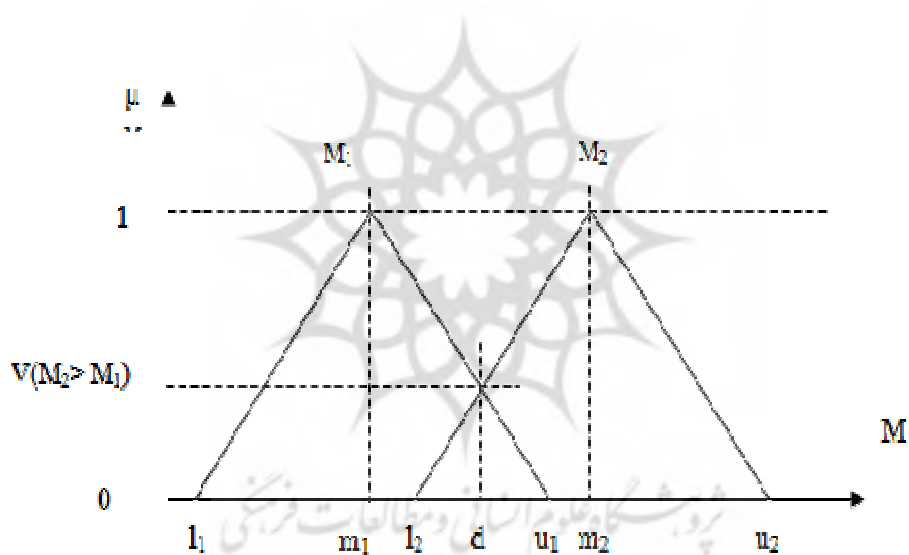
شکل ۱: تقاطع بین M_1, M_2
