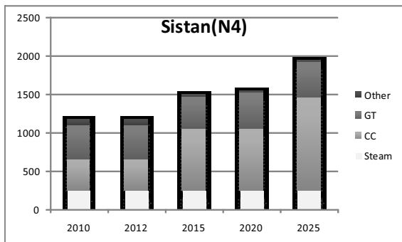
نمودار ۴: ظرفیت نصب شده در منطقه N4
