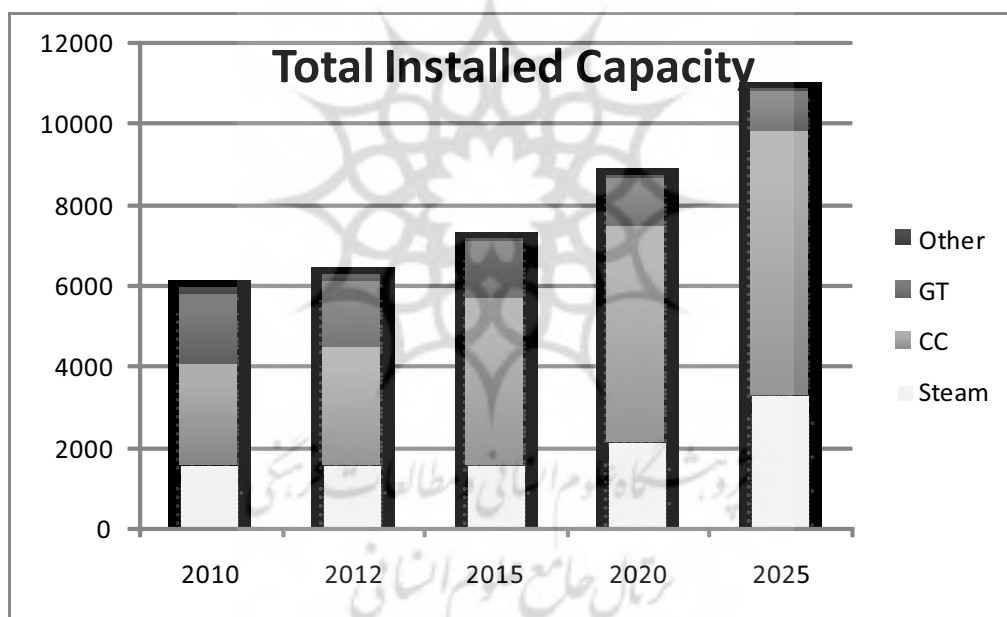
نمودار ۵: کل ظرفیت نصب شده به تفکیک نوع نیروگاه (ارقام بر حسب MW)
