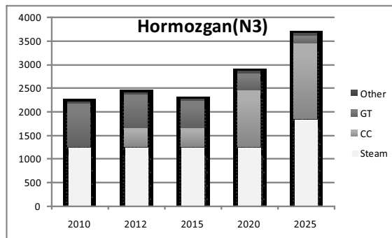
نمودار ۳: ظرفیت نصب شده در منطقه N3
