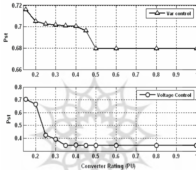
شکل (۱۸): شدت فلیکر در ریتینگ‌های مختلف کانورتر
