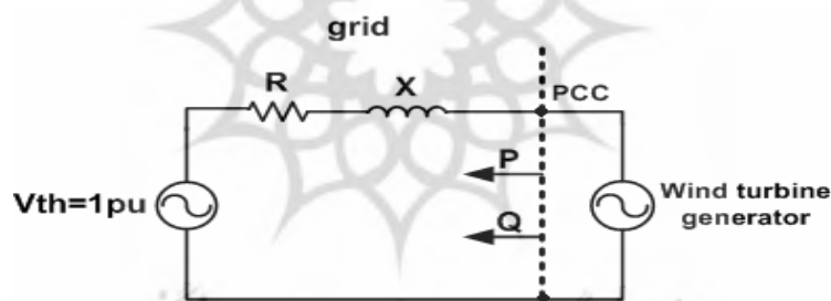
شکل (۱۰): مدار معادل یک توربین بادی متصل به شبکه
