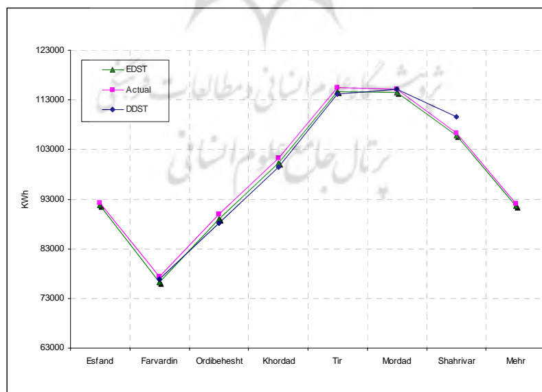
نمودار ۱۲- تغییرات متوسط مصرف روزانه برق در استان تهران ماههای مختلف و سناریوهای مختلف تغییر ساعت - ۶ ماه بهار و تابستان در سناریوهای EDST و DST یکسان است
