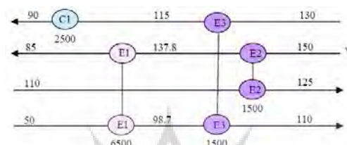
شکل ۸-ب بعد از اصلاح
