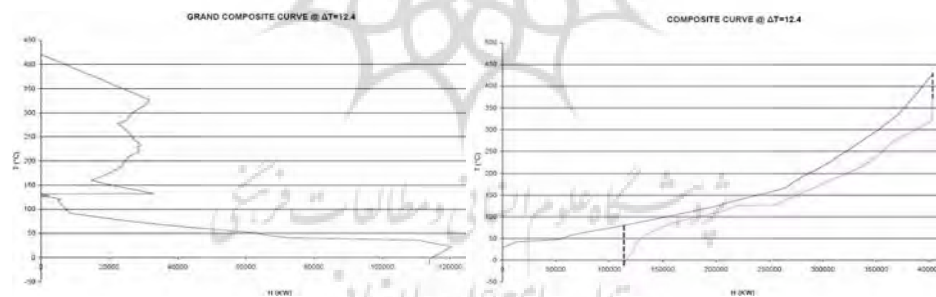
شکل ۱۳- منحنی مرکب کل قبل از اصلاح
