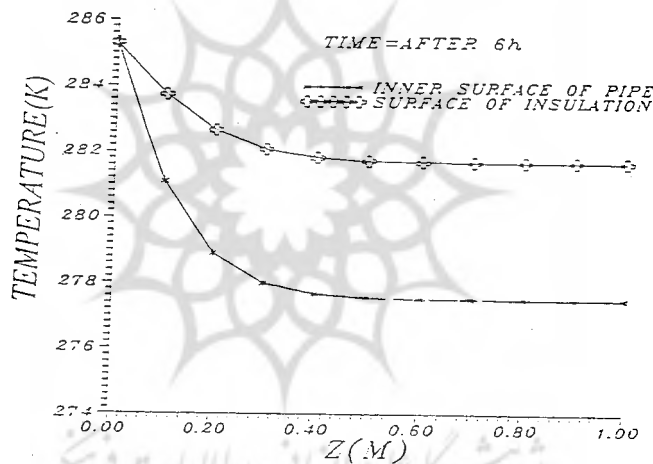
شکل ۵- مقایسه مابین توزیع دمایی از ابتدای امتداد محور شبکه تا انتهای آن برای سطح داخلی لوله واقع بر پرتو شعاعی \theta = 0 درجه و سطح عایق واقع بر پرتو شعاعی \theta = 180 درجه پس از گذشت ۸ ساعت
