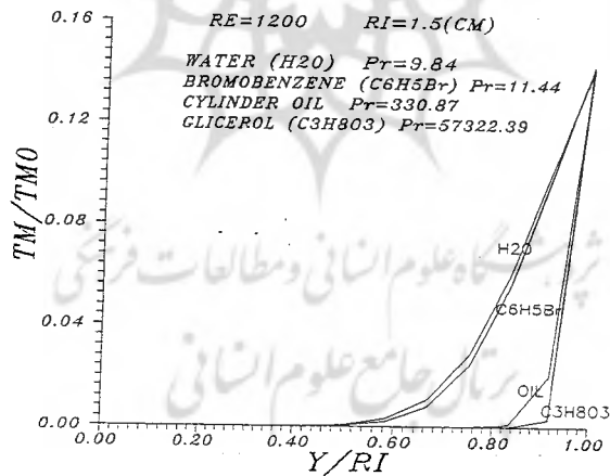
۱۰- نیم پروفیل دمای سیال جاری درون لوله در انتهای امتداد محور شبکه از مرکز لوله تا سطح داخلی لوله واقع بر پرتو شعاعی \theta = 0 درجه برای اعداد پرانتل متفاوت پس از گذشت ۲ ساعت
