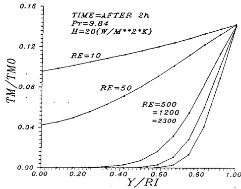
شکل ۹- نیم پروفیل دمای سیال جاری درون لوله در انتهای امتداد محور شبکه از مرکز لوله تا سطح داخلی لوله واقع بر پرتو شعاعی \theta = 0 درجه برای اعداد رینولدز متفاوت پس از گذشت ۲ ساعت
