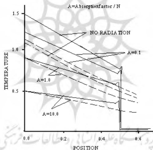
شکل ۳- اثرات شرط مرزی تابش بر هدایت هذلولوی
