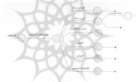
شکل ۳- زیر سیستم تقطیر اتمسفری
