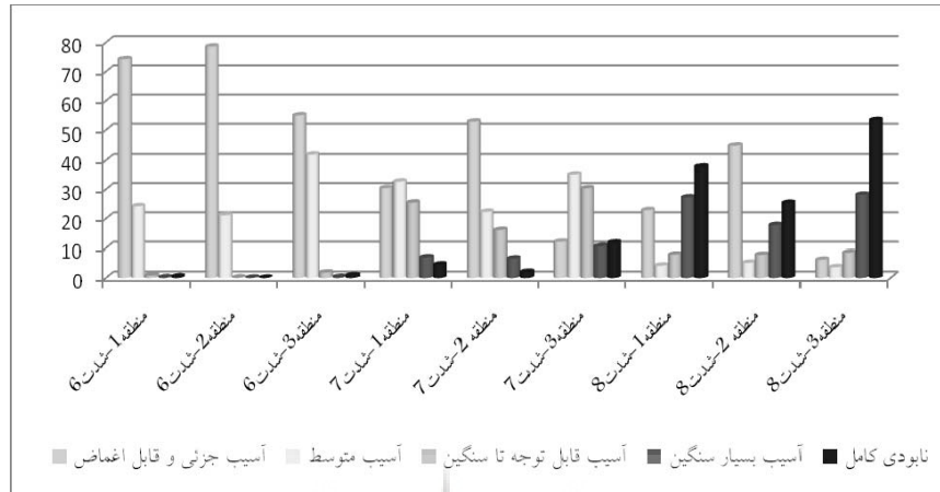
شکل ۵: نمودار میزان آسیب‌پذیری ساختمانی مناطق مختلف شهری زنجان در برابر شدت‌های مختلف زلزله
