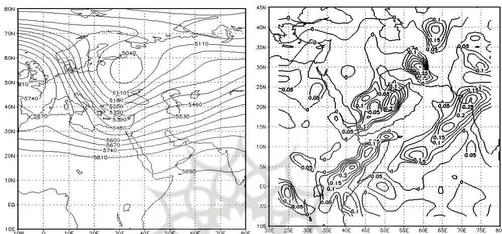
شکل ۱۴: الگوی آرایش پربندی در تراز ۵۰۰
