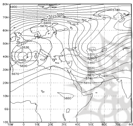
شکل ۱۸: الگوی آرایش پربندی در تراز ۵۰۰
