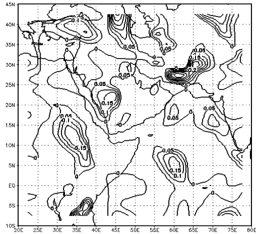
شکل ۵: نقشه‌ی وزش رطوبتی تراز ۸۵۰ هکتوپاسکال روز ۱۳۸۲/۰۹/۱۶
