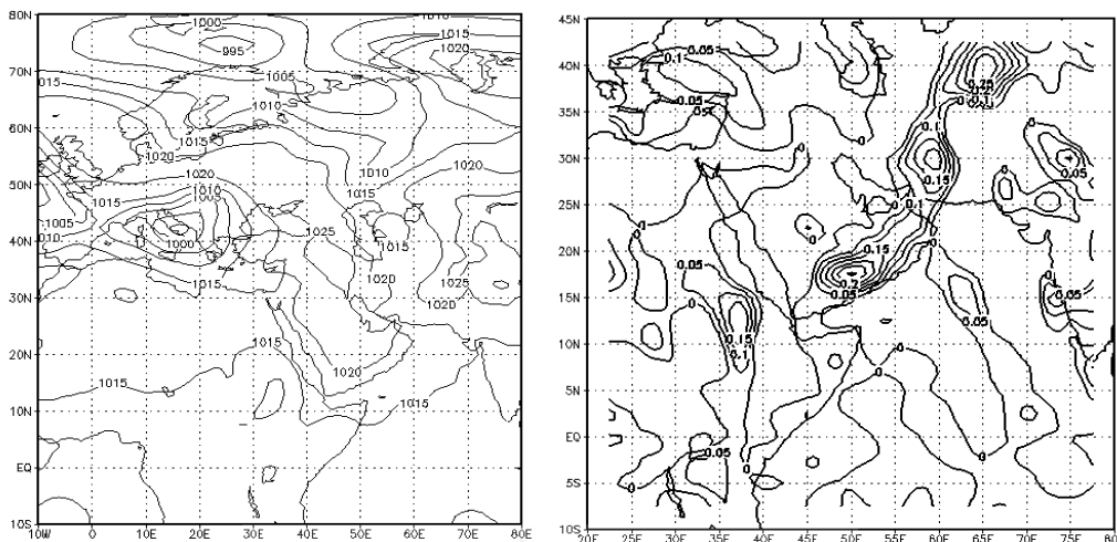
شکل ۳: نقشه‌ی وزش رطوبتی تراز دریا
