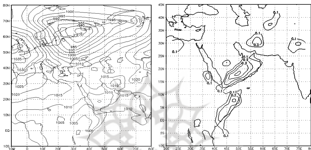
شکل ۱۱: نقشه‌ی وزش رطوبتی تراز دریا
