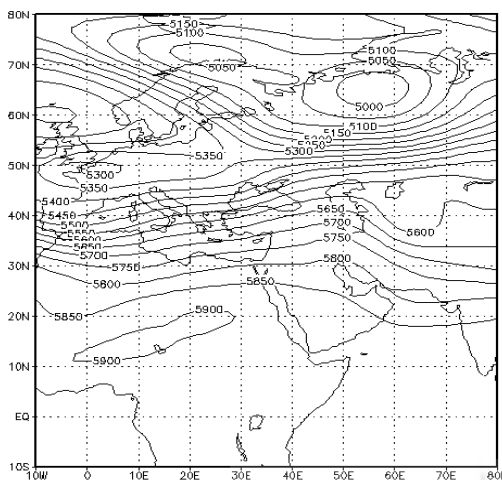
شکل ۶: الگوی آرایش پربندی در تراز ۵۰۰ هکتوپاسکال روز ۱۳۸۲/۰۹/۱۶
