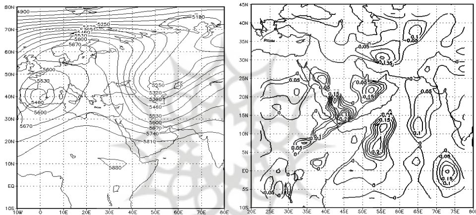
شکل ۱۷: نقشه‌ی وزش رطوبتی تراز ۸۵۰
