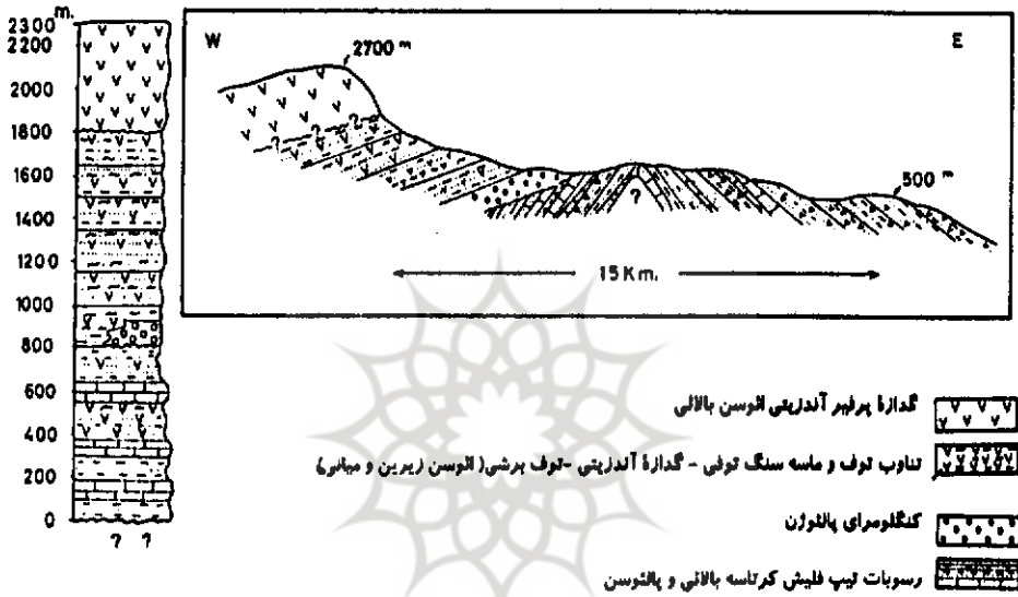
شکل (۲): چگونگی قرارگیری رسوبات کرتاسه، پالئوژن و گدازه‌های ائوسن بالایی در تاقدیس غرب آستارا. (۱۰)
