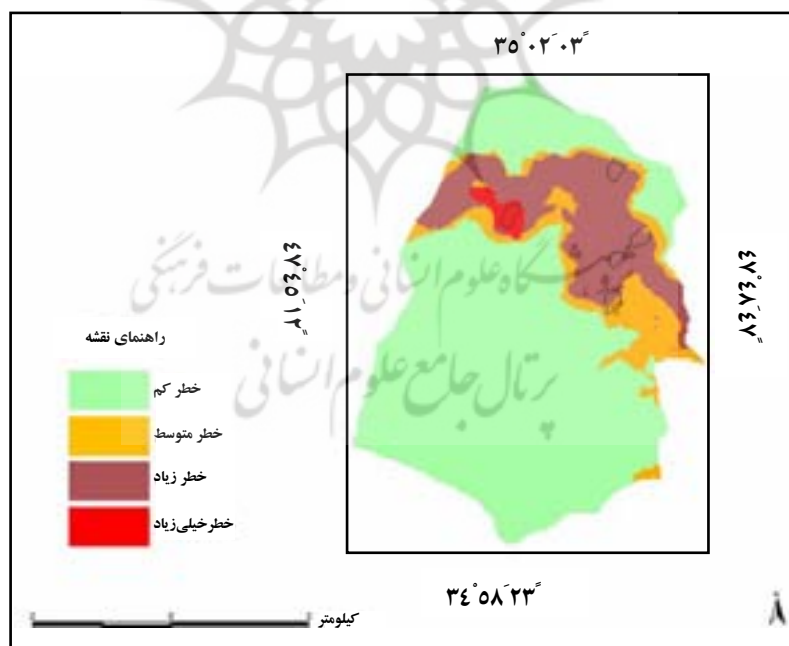
شکل ۵: نقشه پهنه‌بندی خطر زمین‌لغزش حوضه آبریز چرمه به روش ارزش اطلاعاتی مأخذ: نگارندگان
