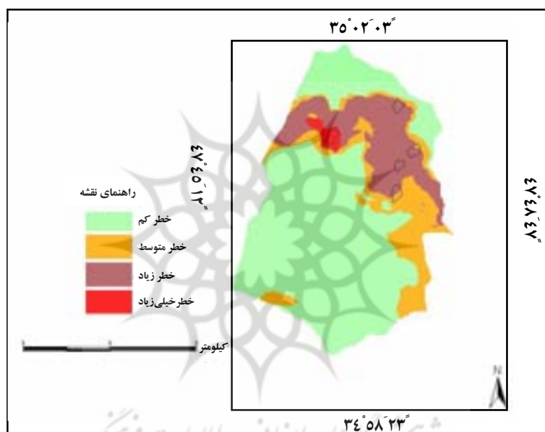
شکل ۳: نقشه‌ی پهنه‌بندی خطر زمین لغزش حوضه‌ی آبریز چرمه به روش تراکم سطح
