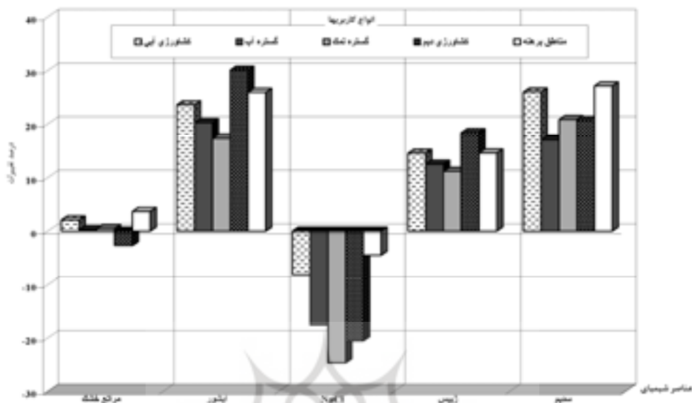
شکل ۳: نمودار فوق درصد تغییرات افزایشی و کاهش مساحت انواع کاربری‌های اراضی منطقه را در محدوده‌ی غلبه عناصر شیمیایی از جمله سدیم، ژپس، آبشور، NaCl و نیز در محدوده مناطق دارای پوشش گیاهی مرتعی از نوع خاص مناطق خشک نشان می‌دهد. چنانکه مشهود است در محدوده غلبه NaCl انواع کاربری‌ها با روند کاهش روبرو شده‌اند.
