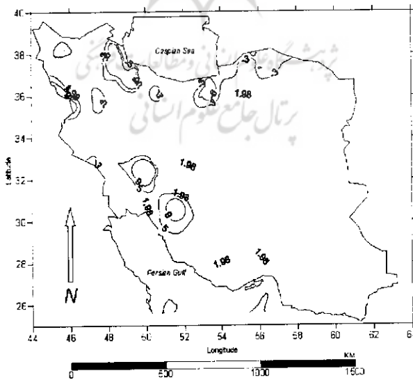
نقشه ۴: میزان تغییرات بارش سالانه‌ی ایران زمین طی دوره آماری ۱۹۶۱-۲۰۰۳
