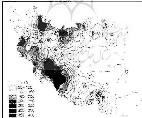
شکل ۷: بارش‌های واقعی زمستان سال ۱۳۷۹ بر اساس اطلاعات دریافتی از ایستگاه سینوپتیک کشور
