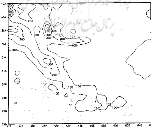
شکل ۵: همانندسازی بارش زمستان ۱۳۷۶ با مدل RegCM3 و طرحواره گزل AS
