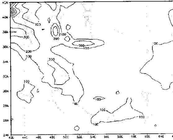
شکل ۴: همانند شکل ۳ اما با استفاده از طرحواره گزل FC
