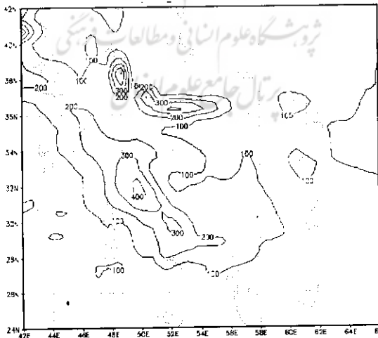
شکل ۹: همانند شکل ۸ اما با استفاده از طرحواره گرل FC
