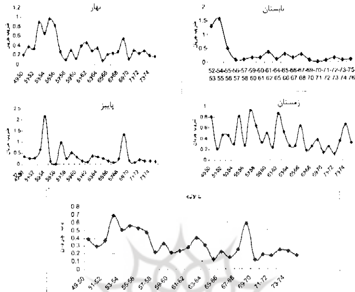
شکل ۴-۲: نمودار ضریب جریان سالانه و فصلی حوضه آبریز سعیدآباد چای ایرانق
