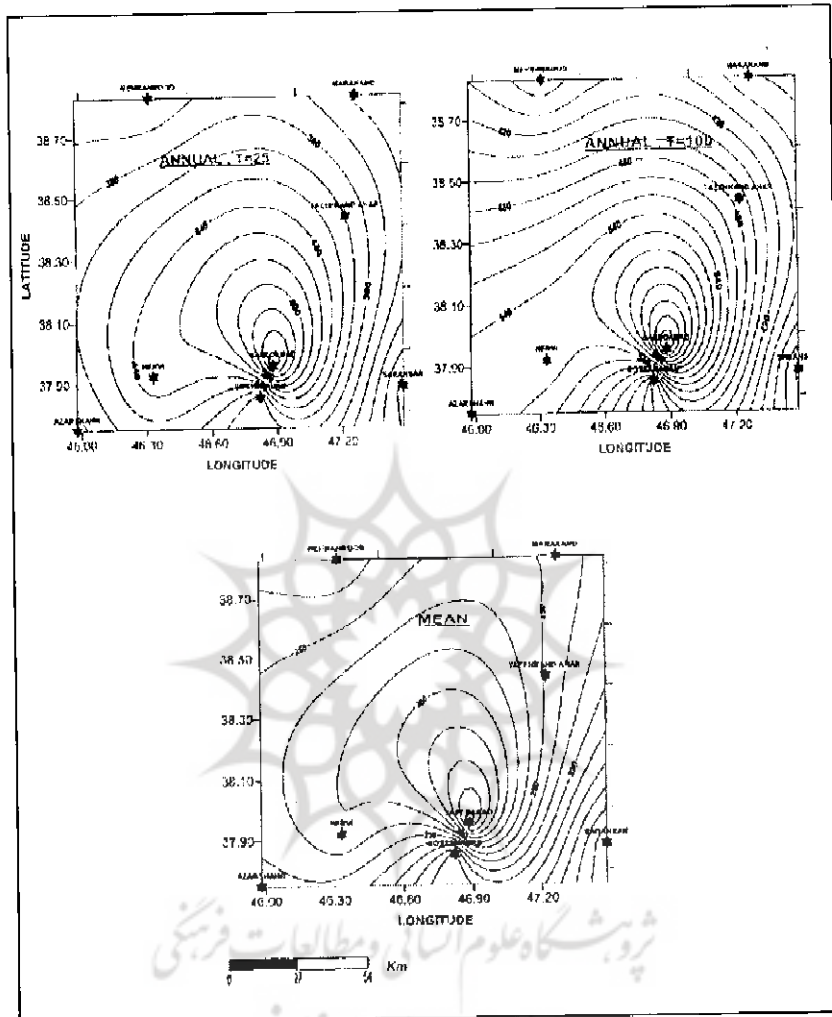
شکل ۲-۳: خطوط همباران سالانه منطقه سعیدآباد بر حسب میلیمتر (متوسط، با دوره برگشت ۲۵ و ۱۰۰ سال)
