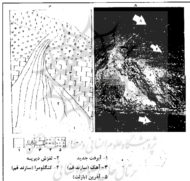
شکل (۱۱-۱): وقوع لغزش دره‌ای در دره آواجیق (B) مقطع تهیه شده از لغزش دره‌ای
