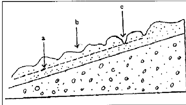
شکل (۱-۱۲) کروکی و برش عرضی لغزش سطحی (a) مسیر جریان آب زیر قشری (b) چاله‌های کوچک در اثر جابه‌جایی مواد ایجاد شده (c) ترک‌های انقباضی
