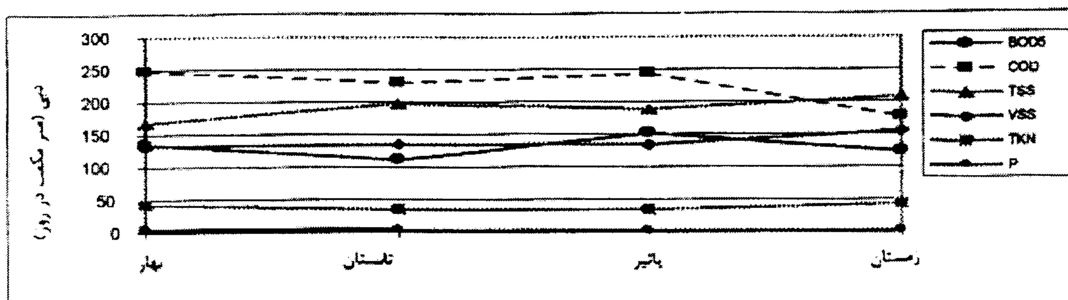
نمودار شماره (۱): تغییرات فصلی غلظت آلاینده های فاضلاب در تصفیه خانه صاحبقرانیه در دوره تحقیق
