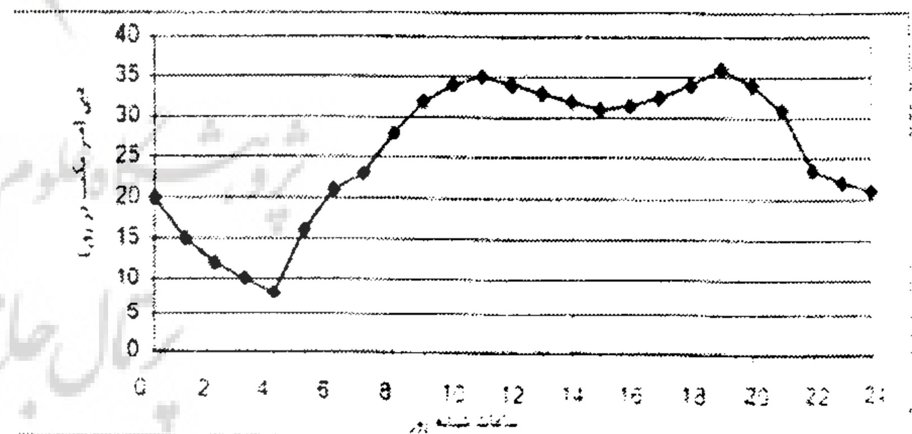
نمودار شماره (۲): میانگین تغییرات ساعتی دبی فاضلاب ورودی به تصفیه خانه صاحبقرانیه در طول دوره تحقیق
