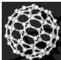
تصویر شماره ۱۳ - مدل ساختار شیمیایی طرح باکمینستر فولر
