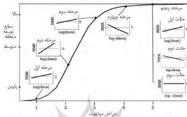
شکل ۲. چهار چوب تئوریک رابطه توسعه و توزیع جمعیت به واسطه مهاجرت خالص
