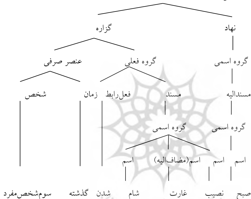
شکل ۱۷: نمودار جمله درونه‌ای (ژرف‌ساخت)
