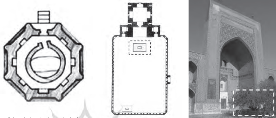
تصویر (۱۱): پلان مزار چلیبی اوغلو، سلطانیه - دوره تیموری. در مزارهای جمالی - جلالی، فضای اطراف مقبره بسیار کوچک است و فضای چندانی جهت گردش زائر در نظر گرفته نشده است. (آرشیو دانشکده معماری دانشگاه علم و صنعت ایران، ۱۳۹۰)
