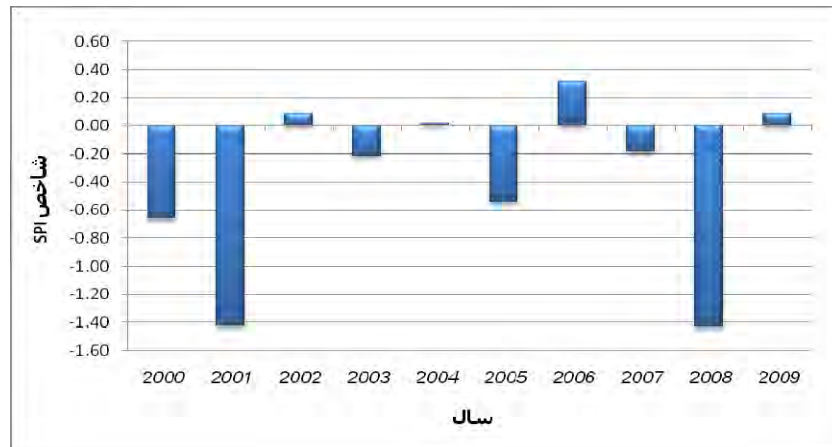
شکل ۱: نمودار میانگین SPI سالانه در استان کردستان طی دوره‌ی آماری ۲۰۰۹-۲۰۰۰
