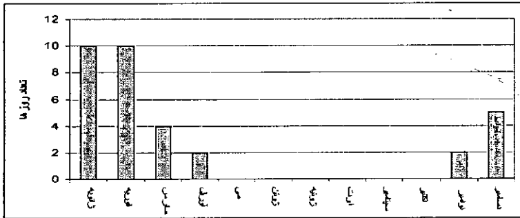
نمودار (۱۴) تعداد روزهای یخبندان در طی سال در ایستگاه دوشان‌تپه (۱۳۴۴-۱۳۷۰)
