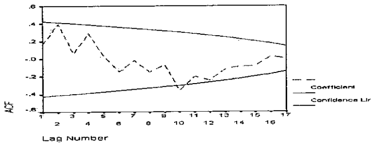
نمودار (۱۱) همبستگی نگار سری زمانی ایستگاه شمال تهران
