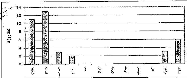
نمودار (۱۶) تعداد روزهای یخبندان در طی سال در ایستگاه ژئوفیزیک (۱۳۷۰-۱۳۸۴)
