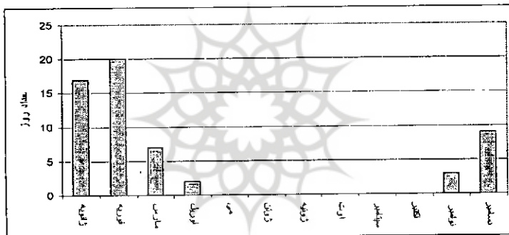
نمودار (۱۲) تعداد روزهای یخبندان در طی سال در ایستگاه شمال تهران (۱۳۸۴-۱۳۶۶)
