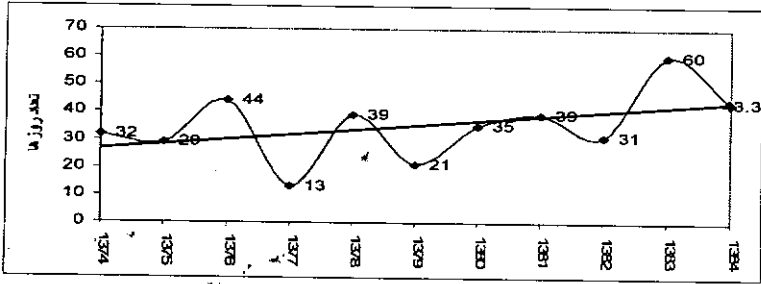
نمودار (۱۷) تعداد روزهای یخبندان ایستگاه جینگر (۱۳۷۴-۱۳۸۴)
