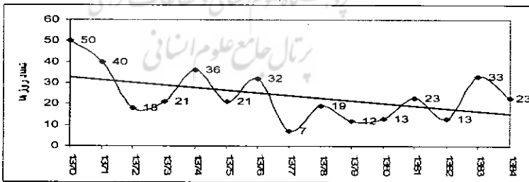
نمودار (۱۳) تعداد روزهای یخبندان ایستگاه دوشان‌تپه (۱۳۷۰-۱۳۸۴)
