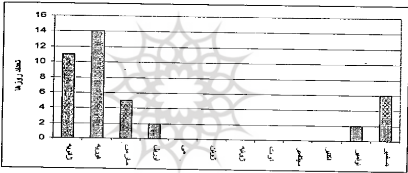
نمودار (۱۸) تعداد روزهای یخبندان در طی سال در ایستگاه جینگر (۱۳۷۴-۱۳۸۴)
