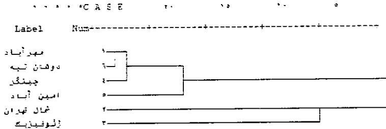
نمودار (۱) درخت خوشه‌بندی دمای شهر تهران
