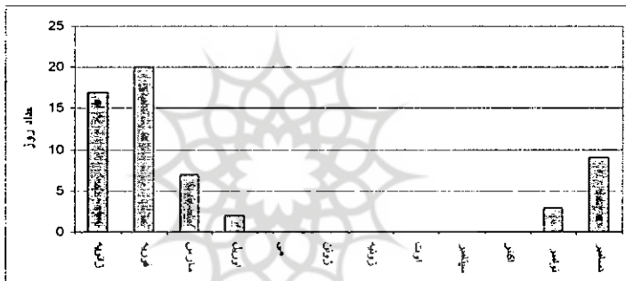
نمودار (۹) تعداد روزهای یخبندان در طی سال در ایستگاه مهرآباد تهران (۱۳۴۴-۱۳۶۴)
