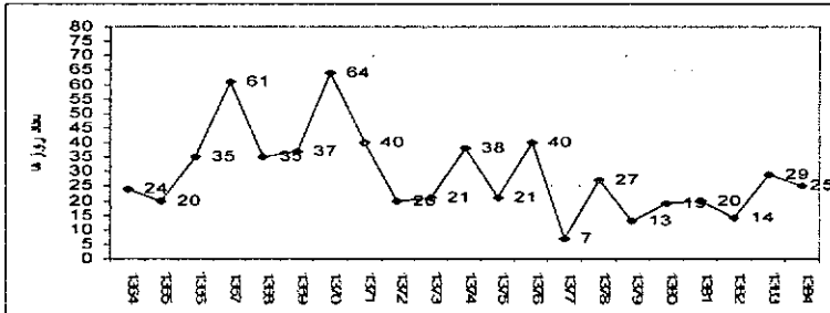
نمودار (۸) تعداد روزهای یخبندان ایستگاه مهرآباد تهران (۱۳۴۴-۱۳۶۴)
