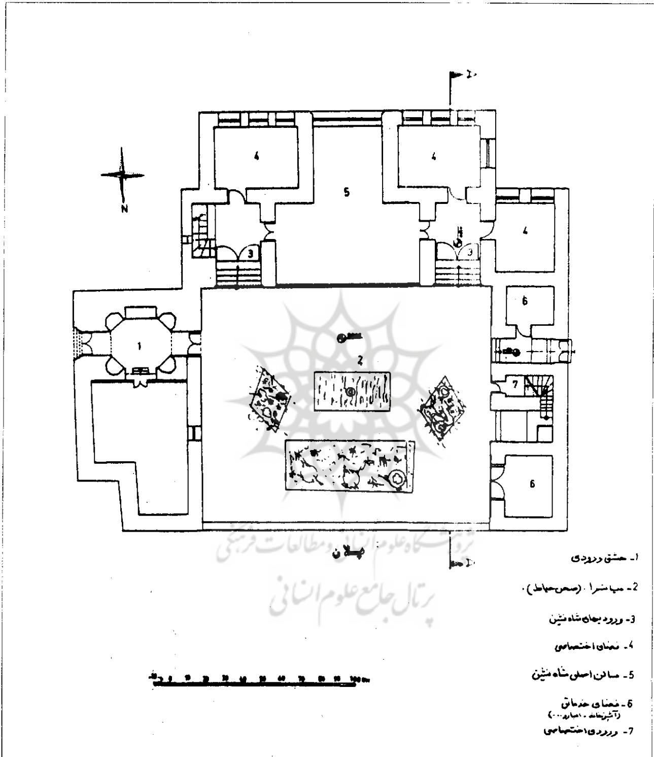
نقشه خانه محمدی - سندج
