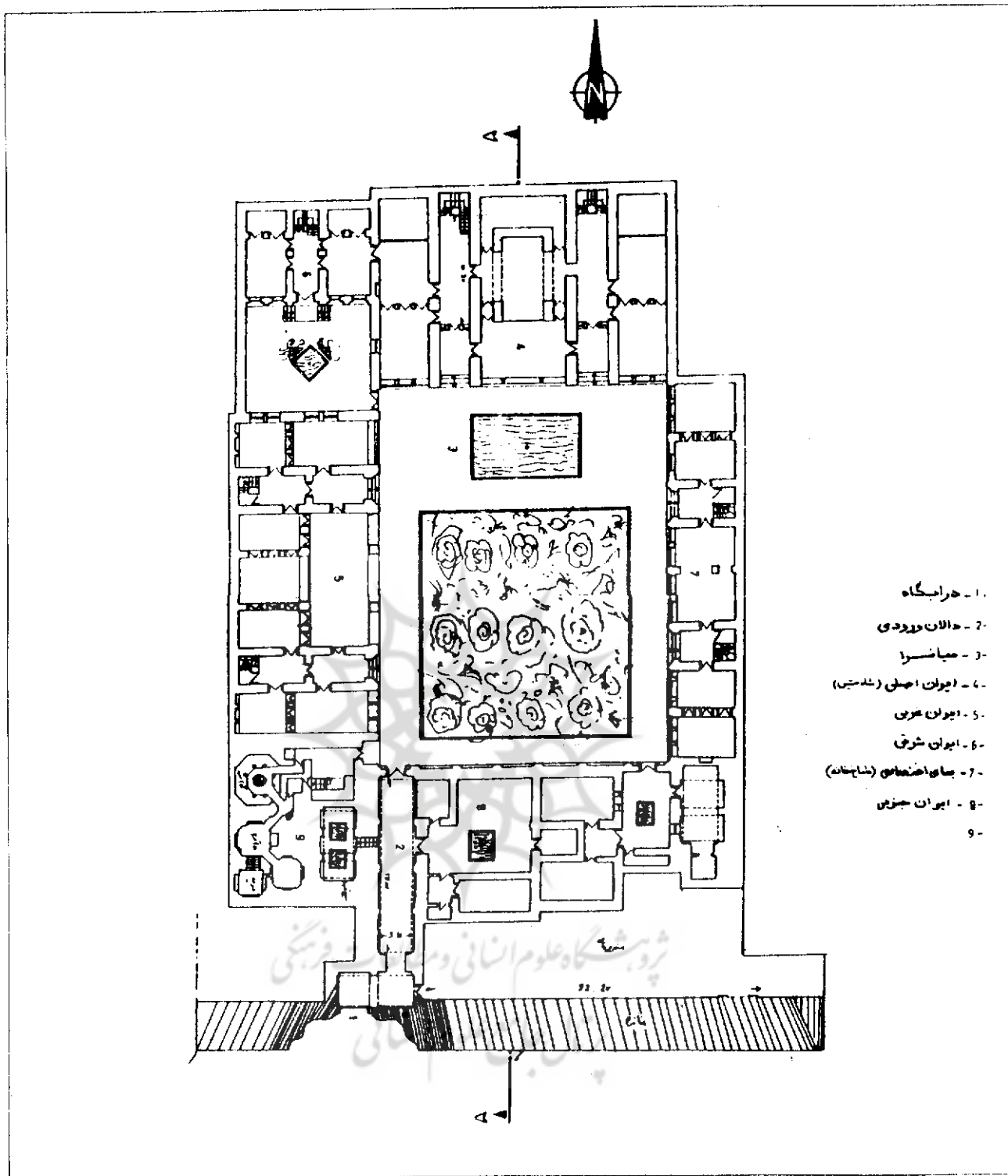
نقشه خانه آصف - سندج
