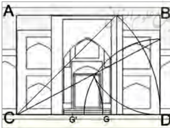
تصویر ۹. ترسیمات هندسی ورودی (نگارندگان)
