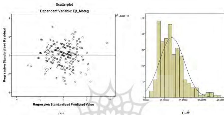
شکل ۱: الف- نمودار هیستوگرام مربوط به توزیع نمرات فاصله مهلبوبایس ، ب- نمودار پراکندگی واریانس‌های استاندارد شده خطاها
