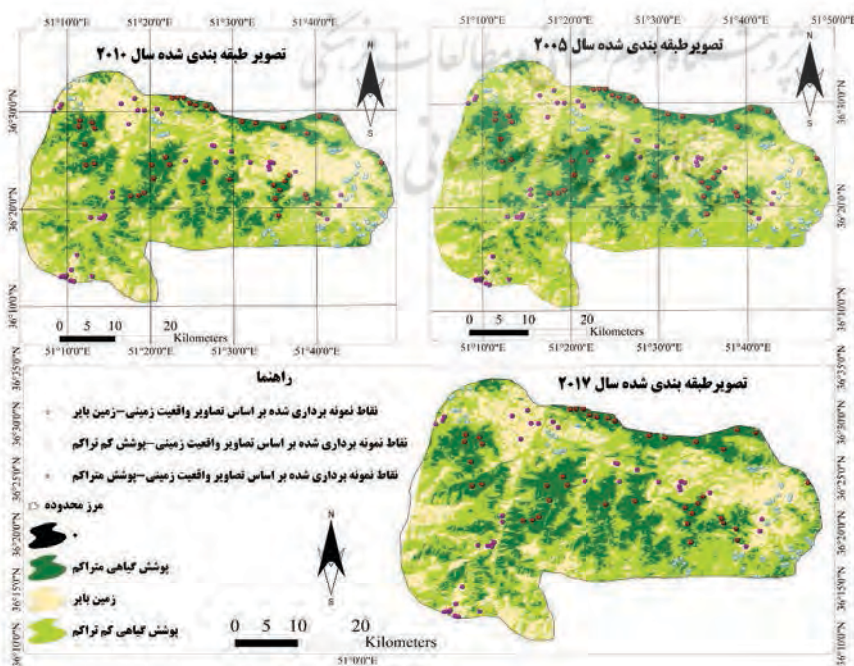
نگاره ۴: کاربری پوشش گیاهی حوزه استان مازندران در بین سال‌های ۲۰۱۷-۲۰۱۰-۲۰۰۵
