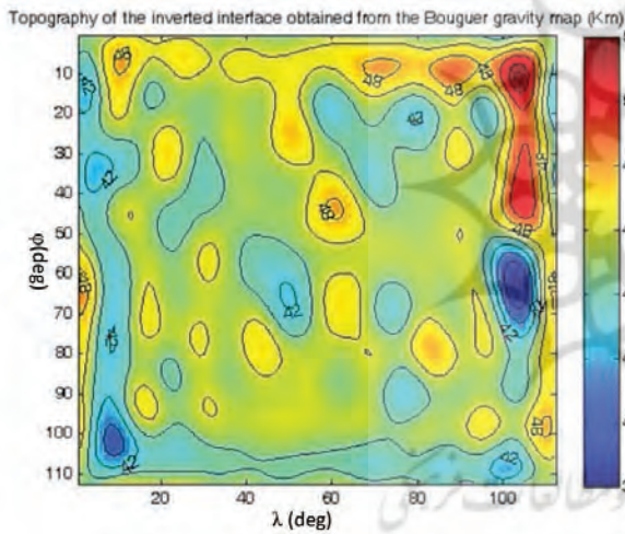
نگاره ۷: عمق موهو بر اساس آنامولی‌های حاصل از داده‌های ثقل‌سنجی NCC (واحد: کیلومتر)
