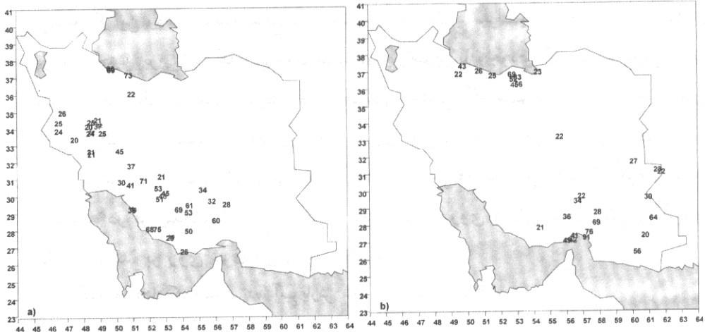
شکل ۱ میزان بارش ۲۴ ساعته بیش از بیست میلی‌متر در روزهای (a) بیست و ششم و (b) بیست و هفتم دسامبر ۲۰۰۴ ( اعداد روی محورها طول و عرض جغرافیائی بر حسب درجه است).
