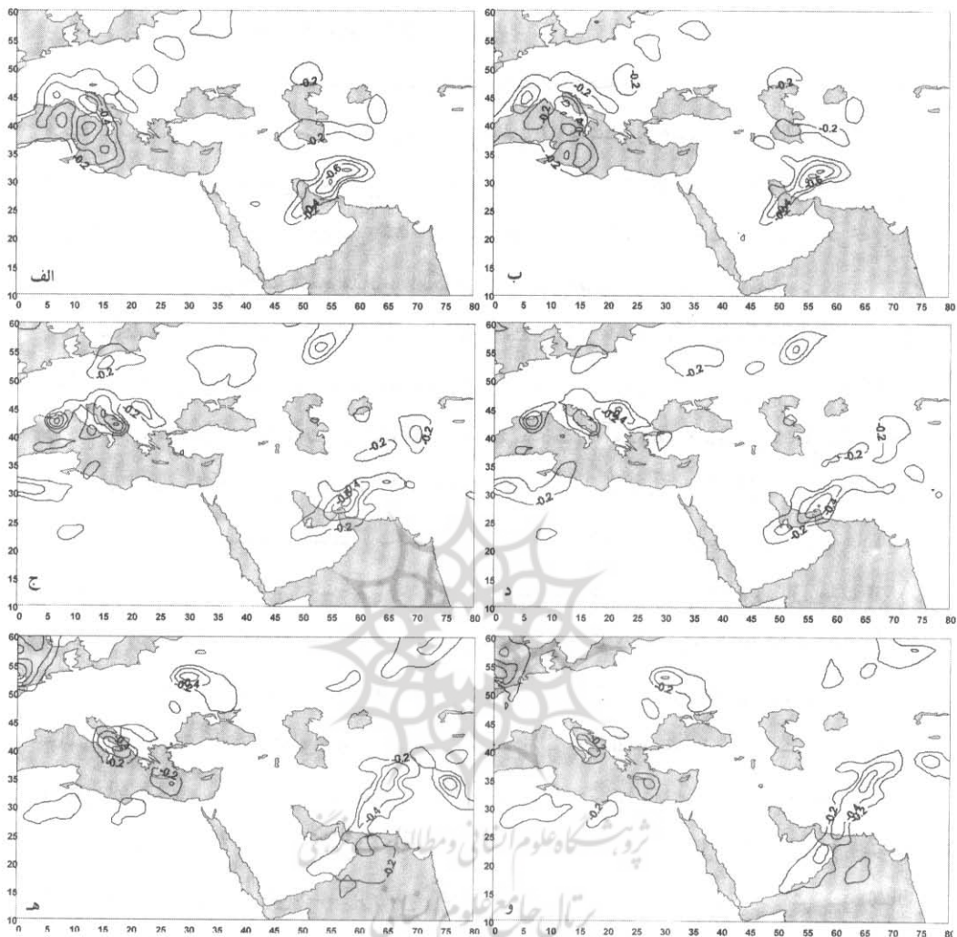
شکل ۴ میدان مؤلفه قائم سرعت باد بالاسو (امگای منفی) در تراز ۵۰۰ هکتوپاسکال برحسب هکتوپاسکال بر ثانیه
