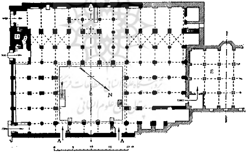
شکل شماره ۷ و ۸ - طرح مسجد جامع دامغان در بالا - و طرح مسجد ناین در پایین (عکس از کتاب هنر ایران تألیف گدار)
