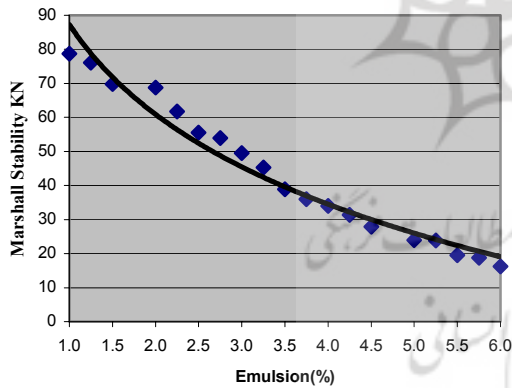
شکل 5 (ز). نمودار تغییرات مقاومت مارشال برحسب درصد امولسیون قیر (3 درصد سیمان)
