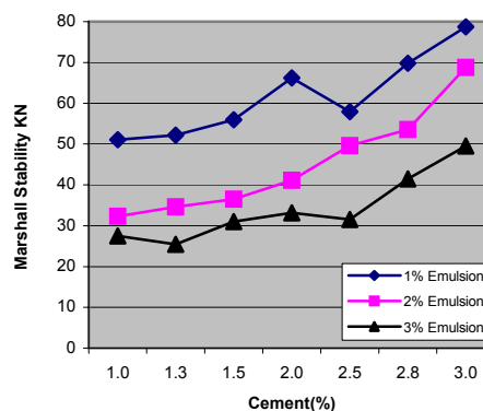
شکل 6 الف. نمودار تغییرات مقاومت مارشال برحسب درصد سیمان (برای 1، 2 و 3 درصد امولسیون قیر)
