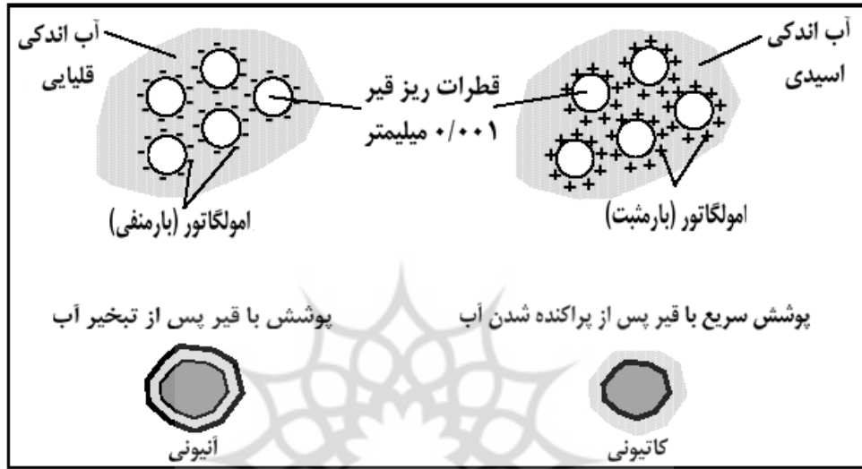
شکل 1. مشخصات امولسیونهای قیر [5]
