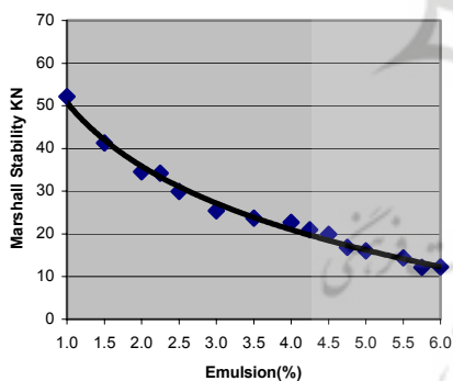
شکل 5 (ب). نمودار تغییرات مقاومت مارشال برحسب درصد امولسیون قیر (1/25 درصد سیمان)
