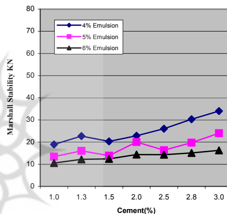
شکل 6 ب. نمودار تغییرات مقاومت مارشال برحسب درصد سیمان (برای 4، 5 و 6 درصد امولسیون قیر)
