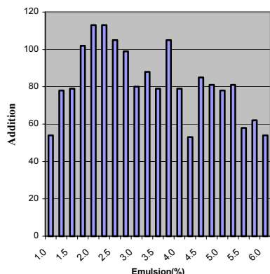
شکل 8. نمودار درصد افزایش مقاومت مارشال به علت استفاده از سیمان برحسب درصد‌های امولسیون قیر مختلف
