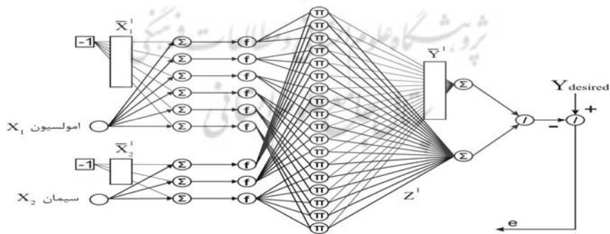
شکل 9. ساختار شبکه عصبی - فازی پیشنهادی با دو ورودی و یک خروجی
