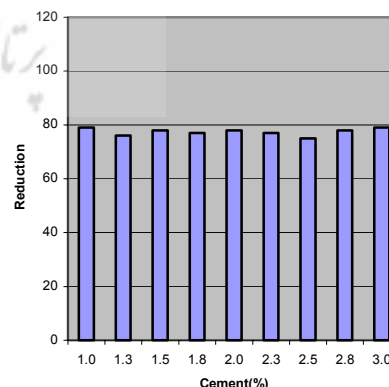
شکل 7. نمودار درصد کاهش مقاومت مارشال به علت استفاده از امولسیون قیر برحسب درصد‌های سیمان مختلف
