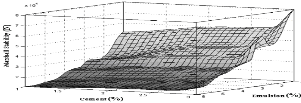
شکل 10. خروجی شبکه عصبی - فازی آموزش دیده
