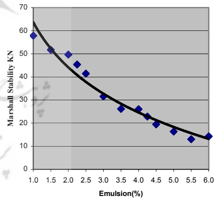
شکل 5 (ه). نمودار تغییرات مقاومت مارشال برحسب درصد امولسیون قیر (2/5 درصد سیمان)
