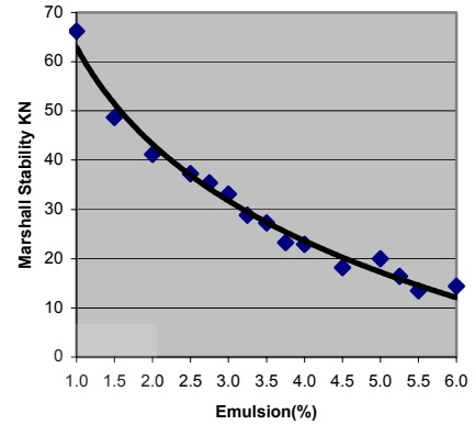
شکل 5 (د). نمودار تغییرات مقاومت مارشال برحسب درصد امولسیون قیر (2 درصد سیمان)
