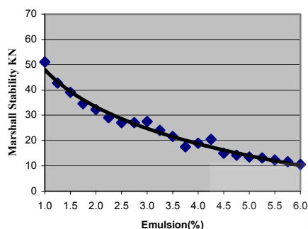
شکل 5 (الف). نمودار تغییرات مقاومت مارشال برحسب درصد امولسیون قیر (1 درصد سیمان)
