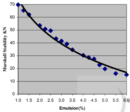
شکل 5 (و). نمودار تغییرات مقاومت مارشال برحسب درصد امولسیون قیر (2/75 درصد سیمان)
