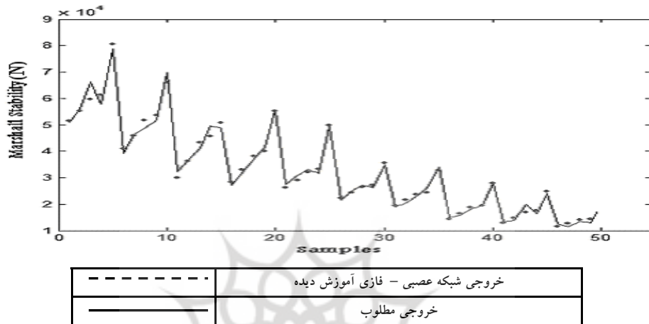
شکل 11. نمودار مقایسه خروجی مطلوب و خروجی شبکه عصبی - فازی آموزش دیده، به ازای داده‌های آزمایش
