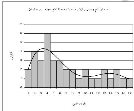
شکل 2. نمودار تابع توزیع ویبول برازش داده شده به تقاطع مجاهدین - ایران
