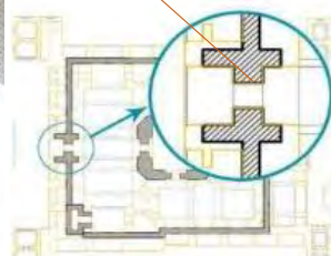
تصویر ۳. پلان گنبدخانه و موقعیت ایوان تیموری. مأخذ: نگارندگان.
