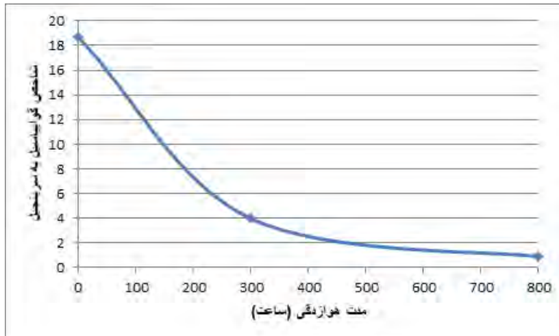
شکل ۵. تغییرات شاخص گوایاسیل به سرینجیل در طول هوازدهی نمونه‌های تیمار نانوآکسید روی
