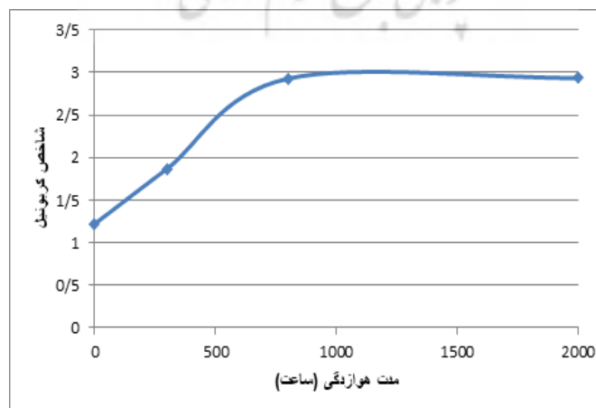
شکل ۳. تغییرات شاخص کربونیل در طول هوازده‌گی نمونه‌های تیمار نانوآکسید روی
