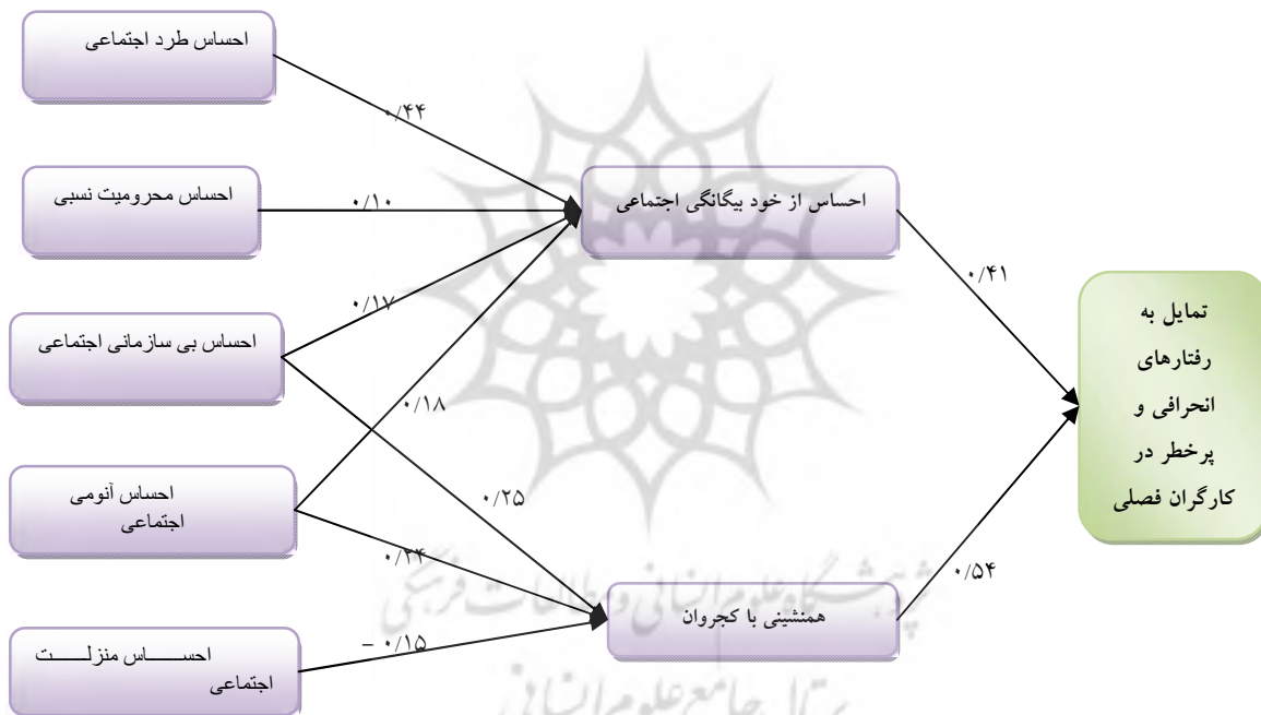
نمودار ۱: مسیر تأثیرگذاری متغیرهای مستقل معنادار در معادله‌ی رگرسیونی بر متغیر وابسته
