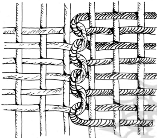
تصویر ۳. حالت قرارگیری تارپود در تکنیک جفت قلاب؛ مأخذ: (Day, 1996, 39)
