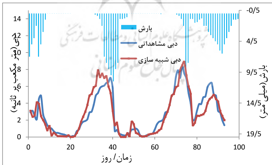
شکل (۶): مقایسه بین جریان اندازه گیری شده و جریان شبیه سازی شده برای دوره اعتبارسنجی (۱۳۹۴/۱۱/۱۳-۱۳۹۴/۰۸/۱۰) Fig (6): Comparison between the measured flow and the simulated flow for the validation period (1394/08/10-1394/11/13)
