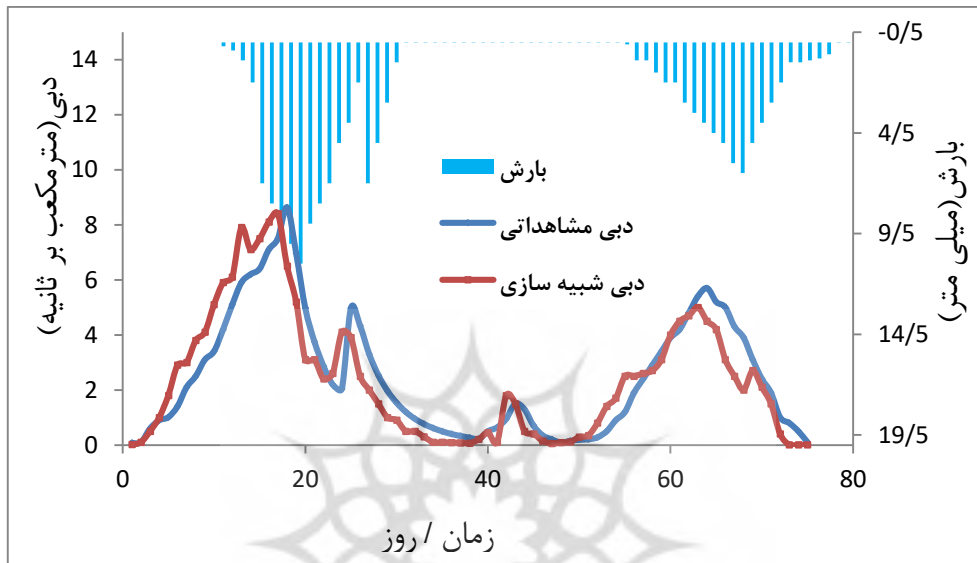
شکل (۵): مقایسه بین جریان اندازه گیری شده و جریان شبیه سازی شده برای دوره واسنجی (۱۳۸۷/۰۹/۱۵-۱۳۸۷/۰۷/۰۵) Fig (5): Comparison between measured flow and simulated flow for calibration period (1387/07/05-1387/09/15)
