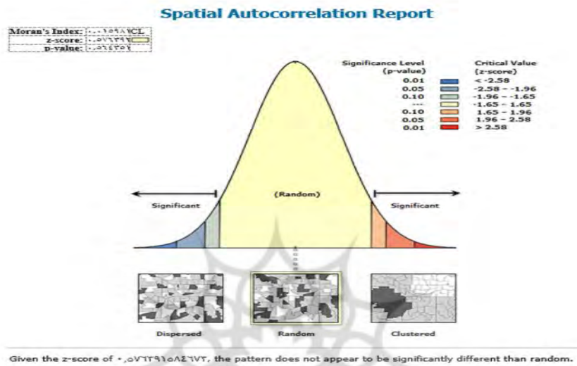
شکل (۶): شاخص موران پارامتر کلر Figure (6): Moran index results for two parameters, chlorine
