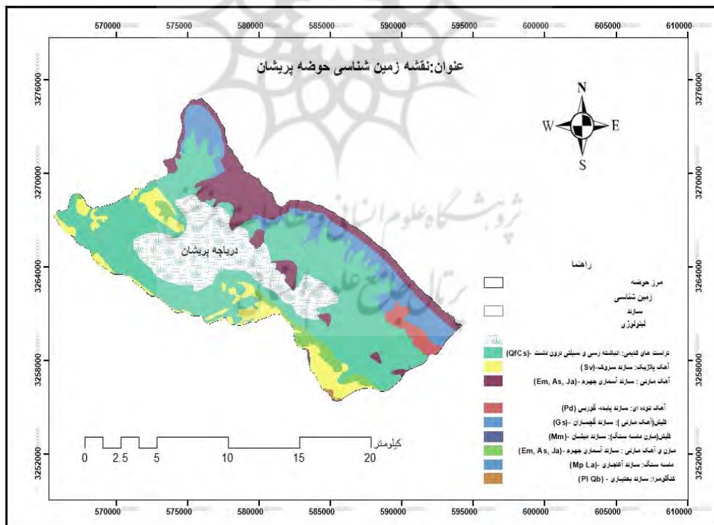
شکل (۲): نقشه‌ی زمین‌شناسی حوضه‌ی پریشان Fig (2): Geological map of Parishan basin
