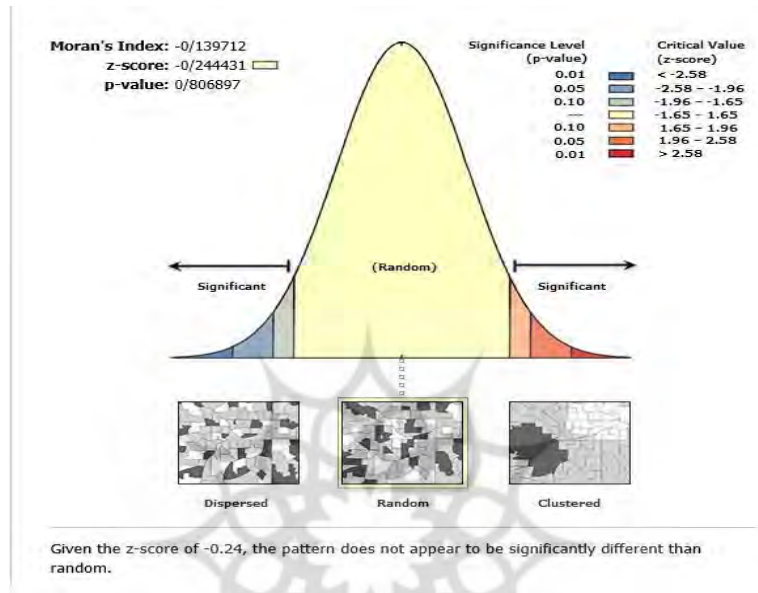
شکل (۴): شاخص موران پارامتر هدایت الکتریکی
