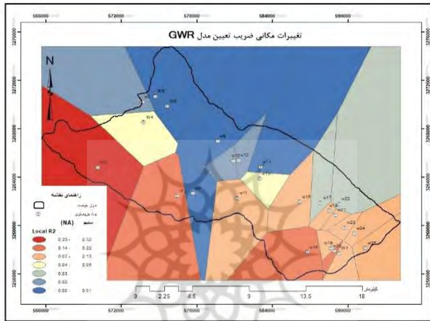
شکل (۱۱): نتایج مدل GWR براساس سدیم
