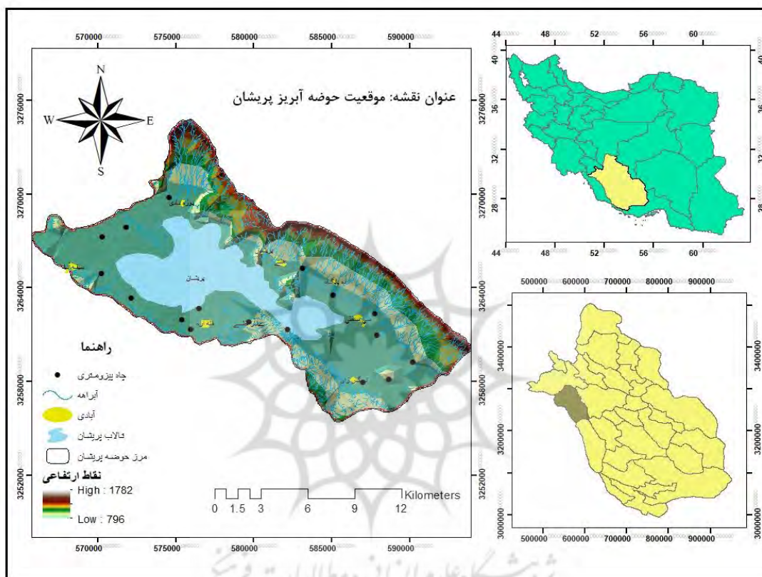
شکل (۱): موقعیت حوضه آبریز پریشان Fig (1): Location of Parishan basin
