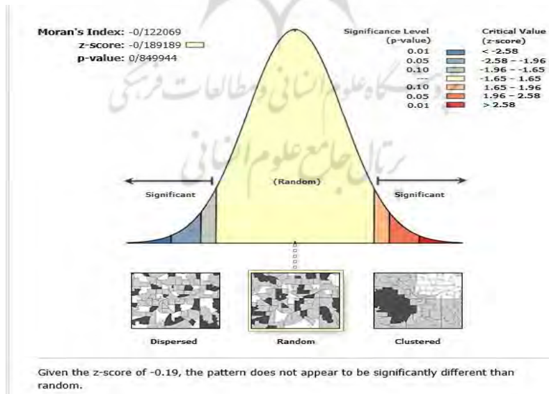
شکل (۵): شاخص موران پارامتر سدیم
