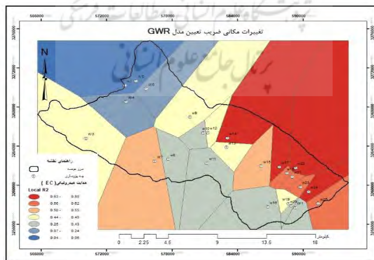
شکل (۸): نتایج مدل GWR براساس هدایت الکتریکی
