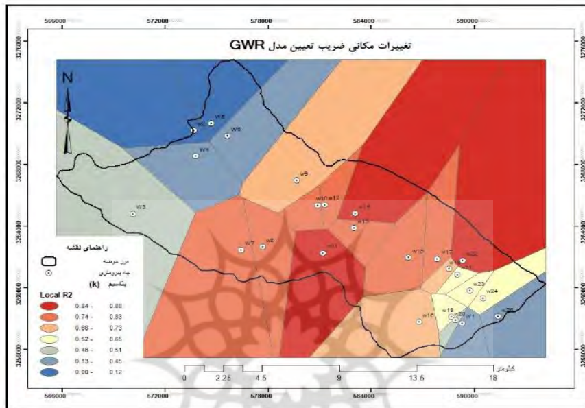
شکل (۹): نتایج مدل GWR براساس پتانسیم Figure (9): The results of the GWR model based on the potassium
