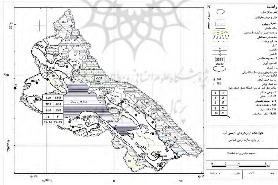
شکل (۳): نقشه‌ی خروجی پارامتر کیفی آب بر روی سازند زمین‌شناسی
