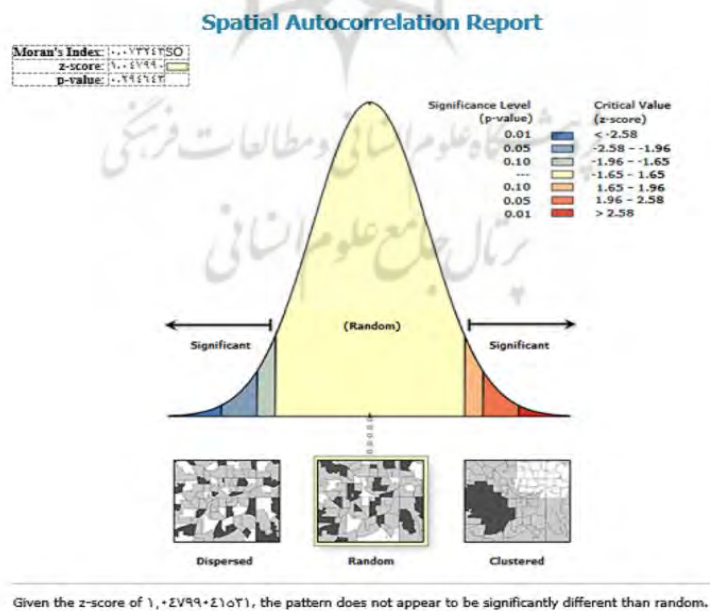
شکل (۷): شاخص موران پارامتر سولفات پتاسیم Figure (7): Moran index of potassium sulfate parameter
