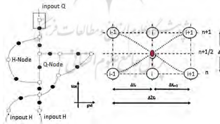
شکل (۳) شبکه‌ی محاسباتی MIKE11 به روش شش نقطه‌ای ابوت برای حل معادلات سنت-ونانت
