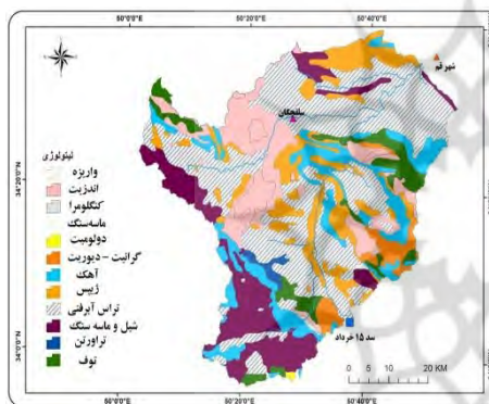
شکل (۵) نقشه‌ی لیتولوژی حوضه
