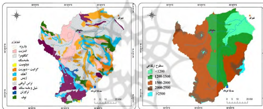
شکل (۴) نقشه‌ی سطوح ارتفاعی حوضه
