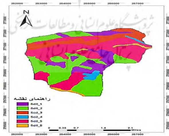
شکل (۴) نقشه‌ی خاکشناسی حوضه‌ی گرین
