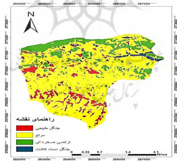
ادامه ی شکل (۳) نقشه ی کاربری اراضی سال ۲۰۰۰
