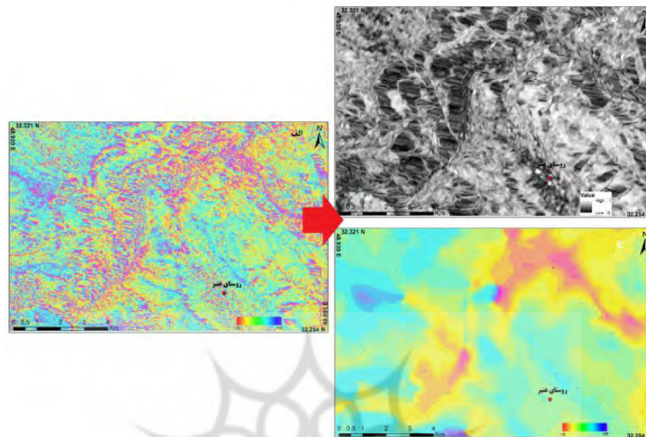
شکل (۴) انجام فیلتر توافقی گلداشتاین بر روی زوج تصویر A_1 از سنجنده ASAR (الف- تداخل نگار فازی مسطح شده ب- تصویر همدوس ج- تصویر تداخل سنجی تفاضلی راداری فیلتر شده)
