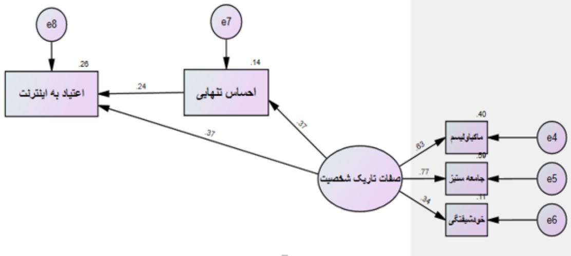
نمودار ۲. مدل نهایی پژوهش و ضرایب استاندارد آن
