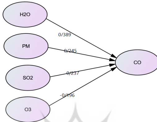
شکل ۸. مسیر متغیرهای تاثیر گذار بر مولکول مونوکسید کربن
