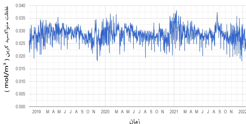
شکل ۱۳. روند تغییرات مونوکسید کربن در بازه زمانی (۱۸-۰۱-۲۲ تا ۱۱-۱۸-۲۰۱۸)،
