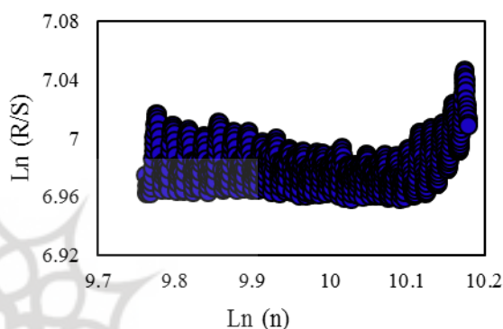
شکل ۵. نمودار پراکنش \ln(R/S) در مقابل \ln(n) الگوی دوم
