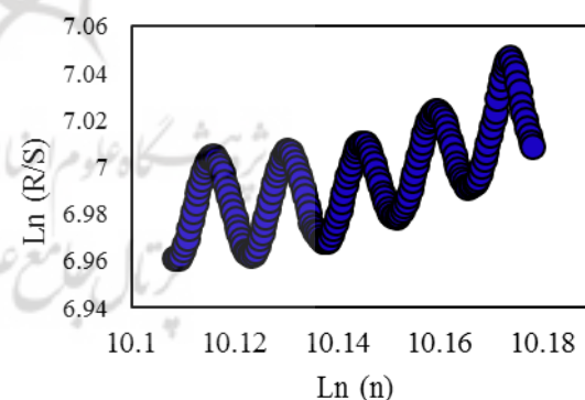
شکل ۷. نمودار پراکنش \ln(R/S) در مقابل \ln(n) بخش دوم الگوی دوم سری زمانی دمای روزانه ایستگاه خرم آباد، منبع: نگارنده، ۱۴۰۲
