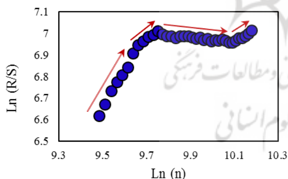
شکل ۷. نمودار پراکنش \ln(R/S) در مقابل \ln(n) بخش دوم الگوی دوم سری زمانی دمای روزانه ایستگاه خرم آباد، منبع: نگارنده، ۱۴۰۲
