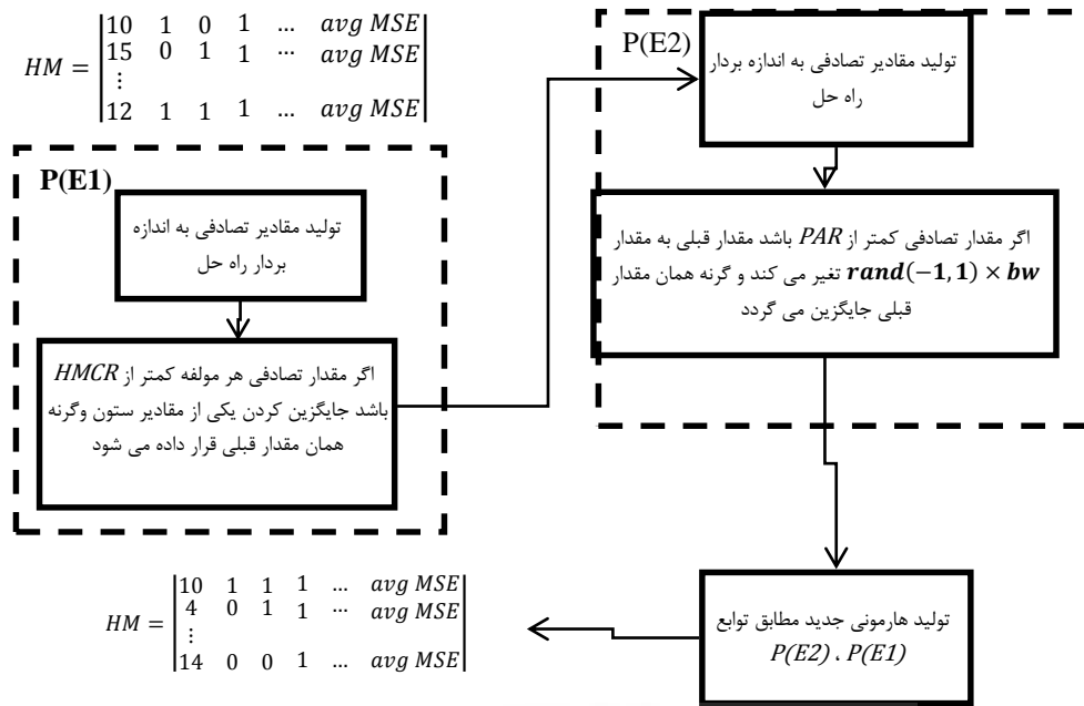
شکل ۳: مفهوم ایجاد هارمونی جدید برای مدل پیش‌بینی پیشنهادی
